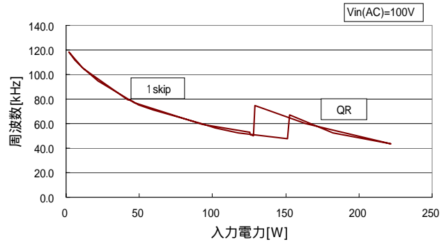
STR-W6700 入力電力-周波数
