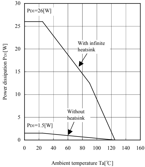
IRIS-G5624A MOSFET Ta-P D1 Curve
